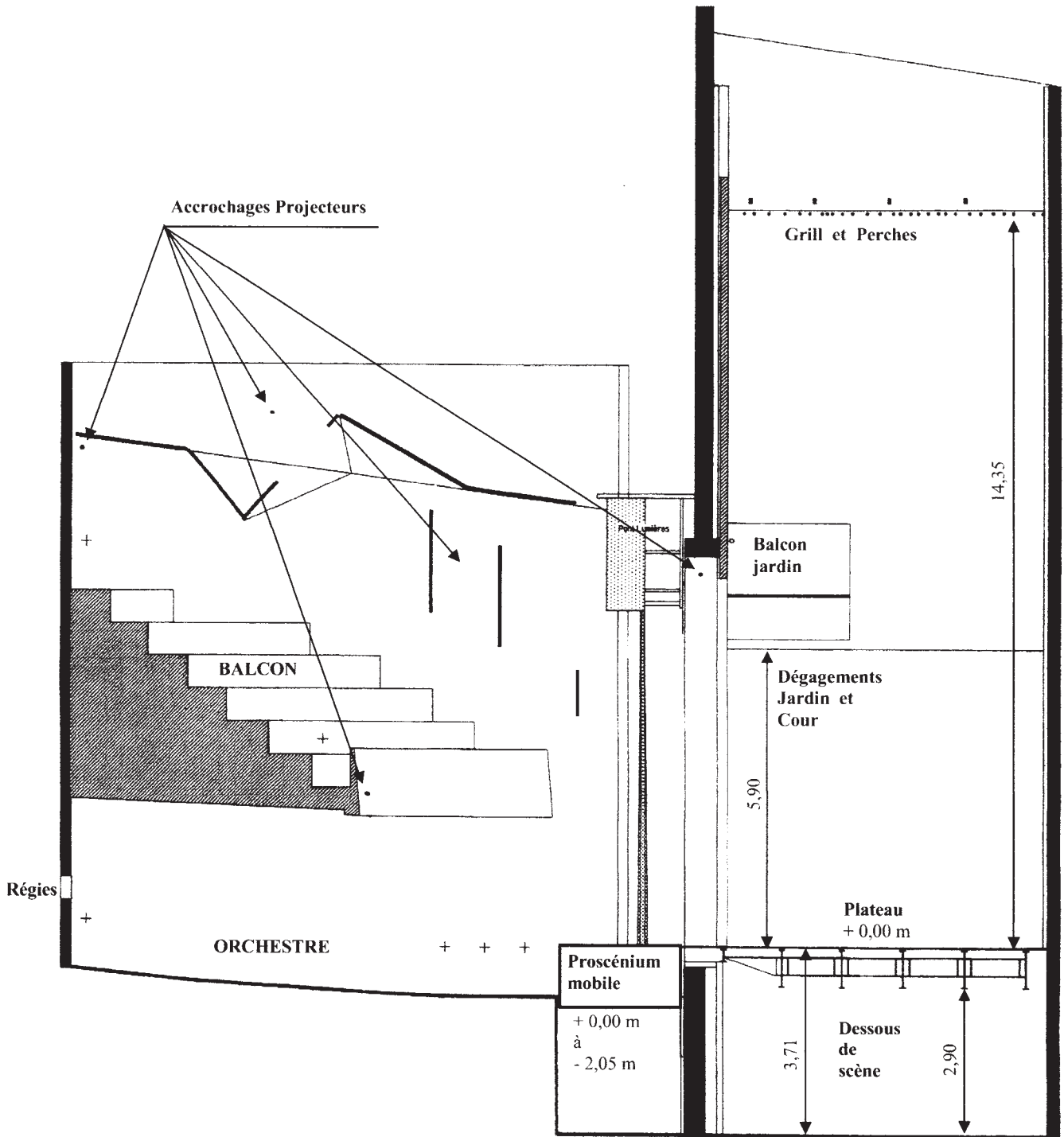
THEATRE SORANO COUPE Salle et cage de scène
